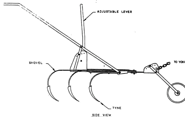
Junior hoe
